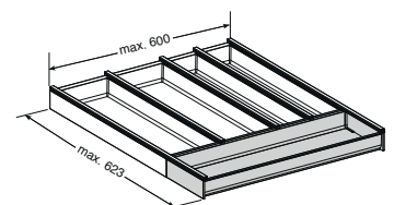
Verlängerungsprinzip (mm)
