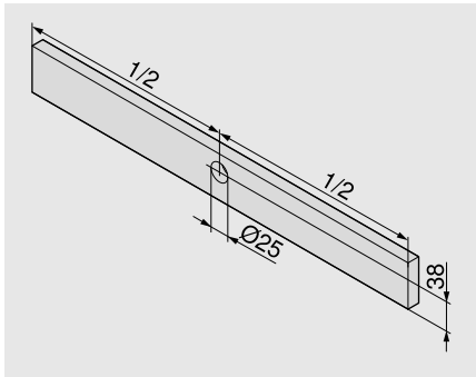
Bohrung Frontblende | Drilling front | Perçage bandeau de la face | Foratura frontale di copertura | Frontal de perforación | Wiercenie pod blendę
