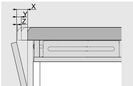
APÜ = Arbeitsplattenüberstand | Worktop overlay | Débord du plan de travail | Sormonto del piano di lavoro | Mesa de preparación de recubrimiento | Wymiar wystającego blatu roboczego
