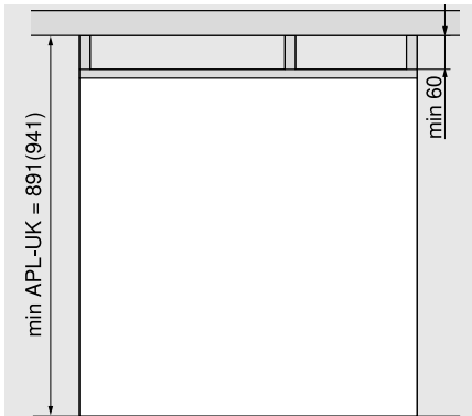
Mindestabstände Arbeitsplatten-unterkante | Minimum distance bottom edge work top | Distances minimales arrête du plan de travail | Distanze minime del bordo inferiore del piano di lavoro | Distancia mínima del borde inferior de la superficie de trabajo | Minimalny odstęp dolnej krawędzi blatu roboczego
