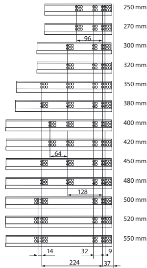
Lochbild 560H Vollauszug 30 KG
