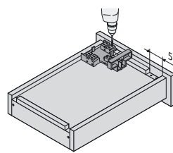
Schubkasten-Bohrlehre (Kupplung)
