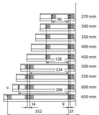
Lochbild 550H Teilauszug 30 KG
