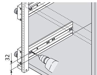
Stangenbohrlehre (Korpusschienenbohrlehre T65.5050 kann auch einzeln bestellt werden)
