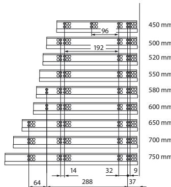
Lochbild 566H Vollauszug 50 KG
