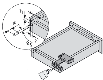
Schubkasten-Bohrlehre (Haken)
